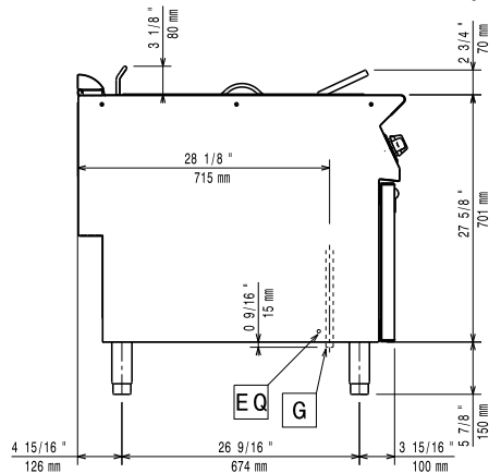
Zij aanzicht
